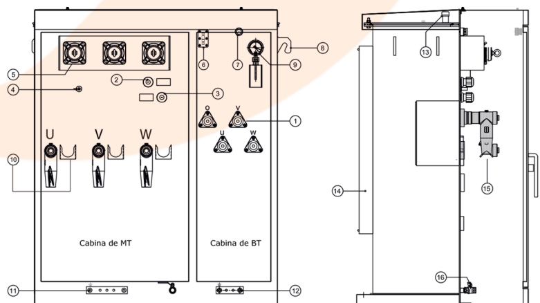
VISTA FRONTAL SIN PUERTAS
